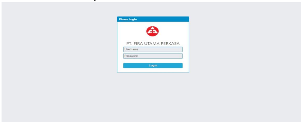
Fig 3: Tampilan Login
